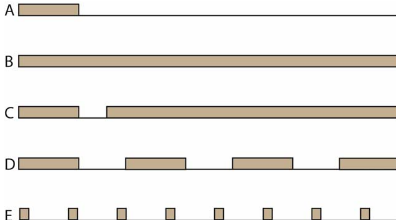
Bild 8: Blinkmuster der Service-LED
