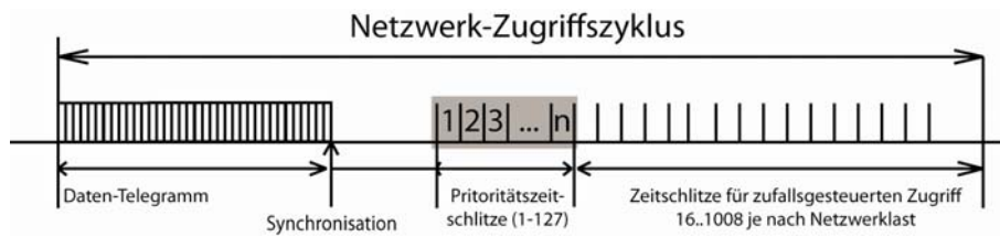
Bild 4: Prioritätszeitschlitz
