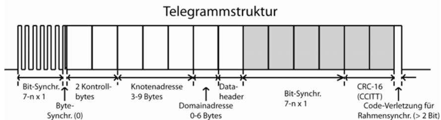
Bild 3: Datenformat
